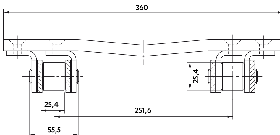
1/2 VUE MAILLON EXTÉRIEUR
