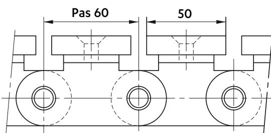
1/2 VUE MAILLON EXTÉRIEUR
