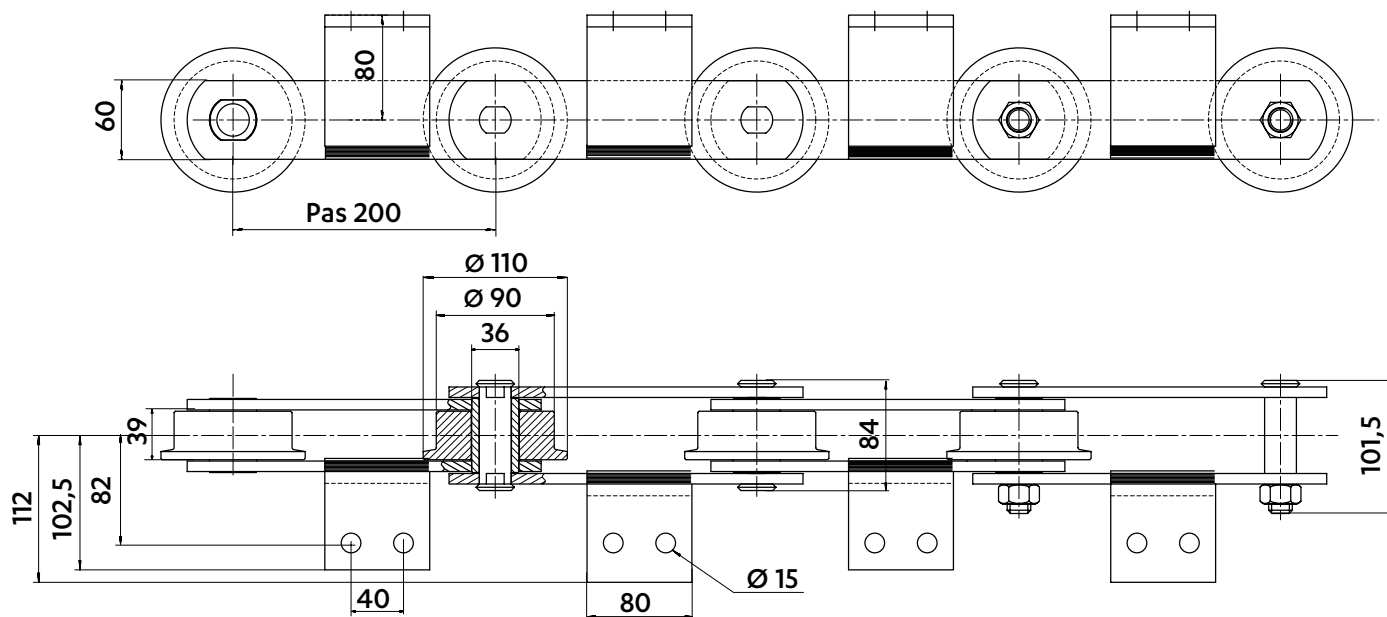
Tablier à deux chaînes en parallèle
