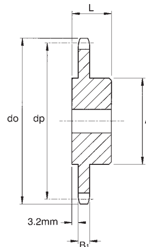
Simplex Sprocket
